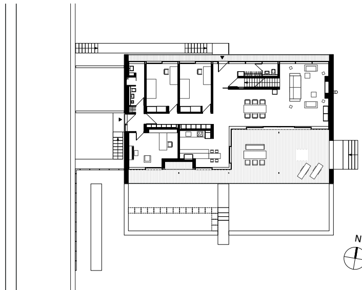
Erdgeschoss mit Aussenanlagen
